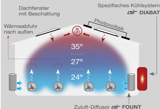
Nachher - mit perfect air naturecooled Lüftungskonzept
